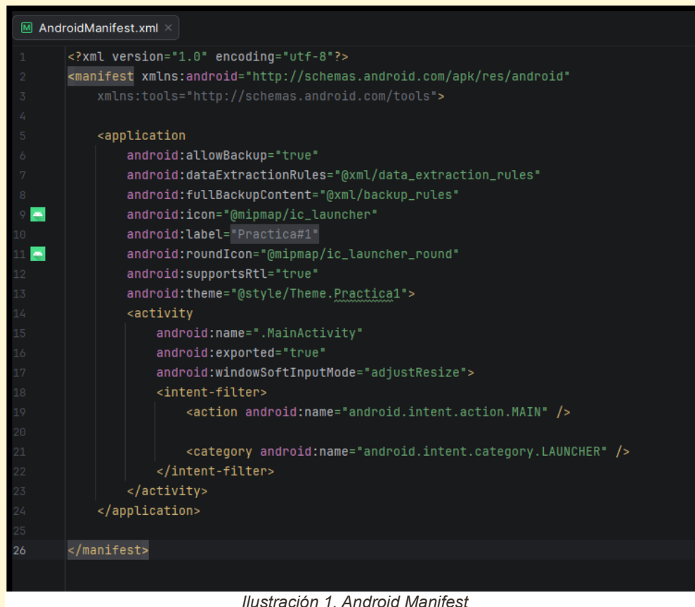
Ilustración 1. Android Manifest
